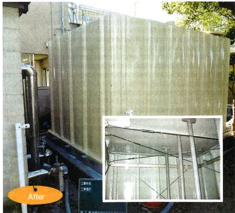
内外にFRPライニングで破断箇所補修後、塗装仕上げ。内部には補強材を取り付け。外観は新品同様に仕上がりに、十分な強度を確保した。
